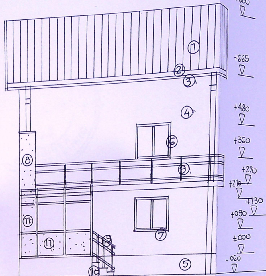
FATADA SUD
