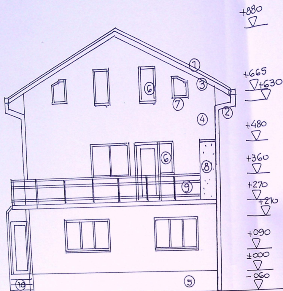
FATADA EST
