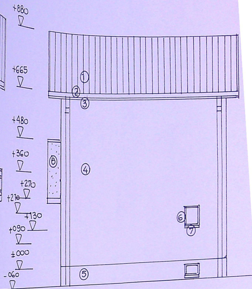
FATADA NORD
